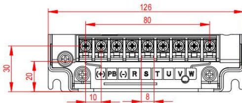
图 4-7 0.75KW ~ 2.2KW 主回路端子示意图
