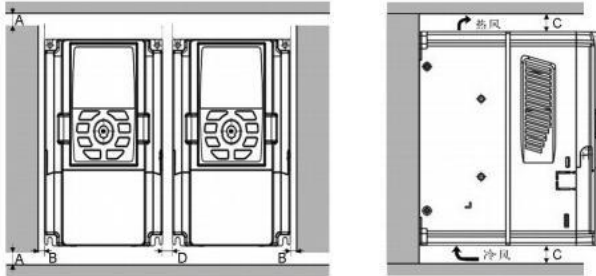
图4-3 并行安装
