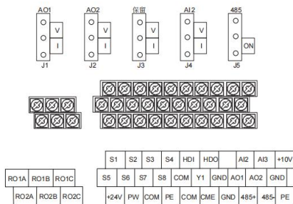
图 4-20 380V 018G/022P 及以上控制端子
