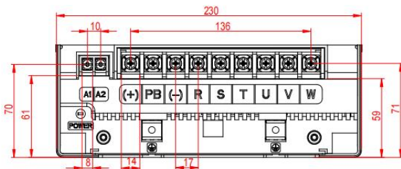
图 4-9 11KW ~ 18.5KW 主回路端子示意图
