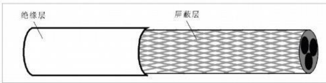
电缆剖面
