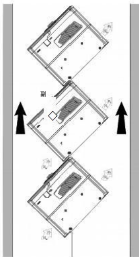
图 4-5 倾斜安装
