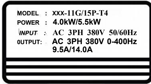
图3-3产品铭牌
