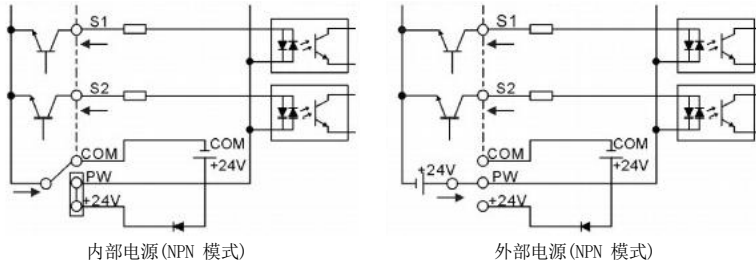
图4-22 NPN模式示意图
