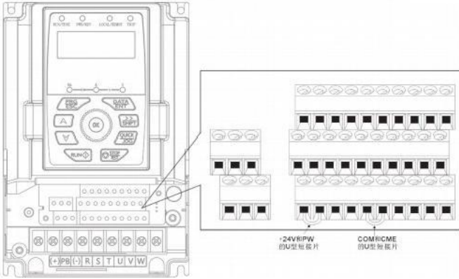
图4-21 U型短接位置示意图
