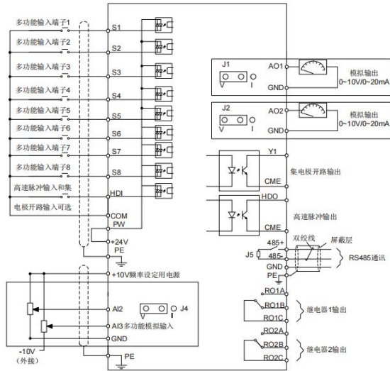
图 4-18 控制回路接线图
