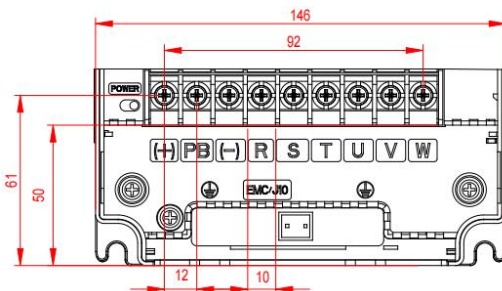
图 4-8 4.0KW ~ 7.5KW 主回路端子示意图
