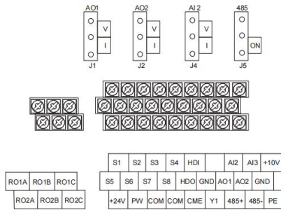
图4-19 380V 015G/018P 及以下控制端子
