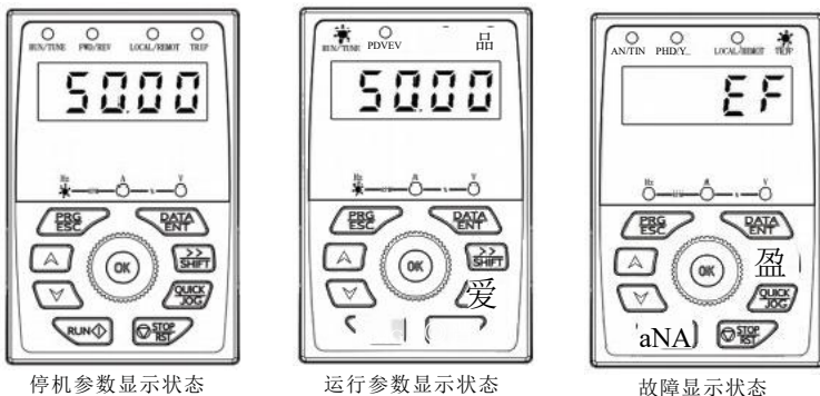
图5-2 状态显示示意图
