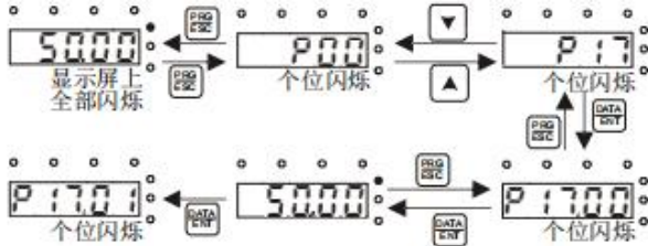
图 5-5 查看参数
